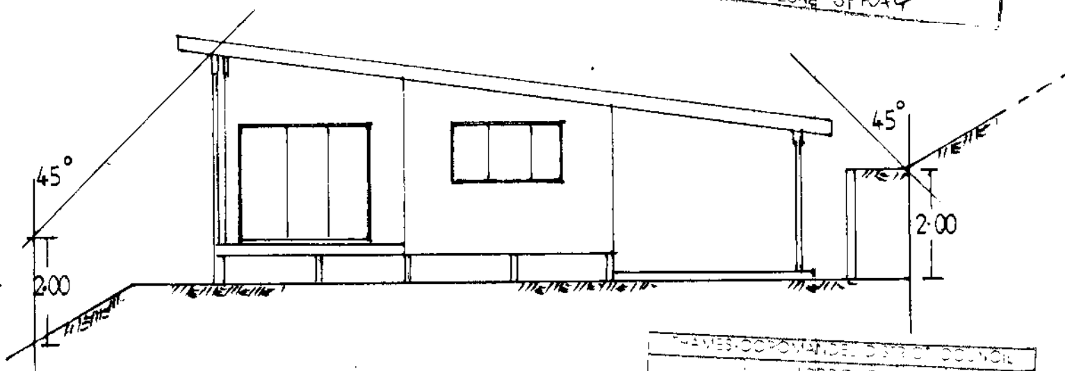
N.W. Elev.
